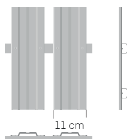
blacha ocynkowana 0,5 mm
